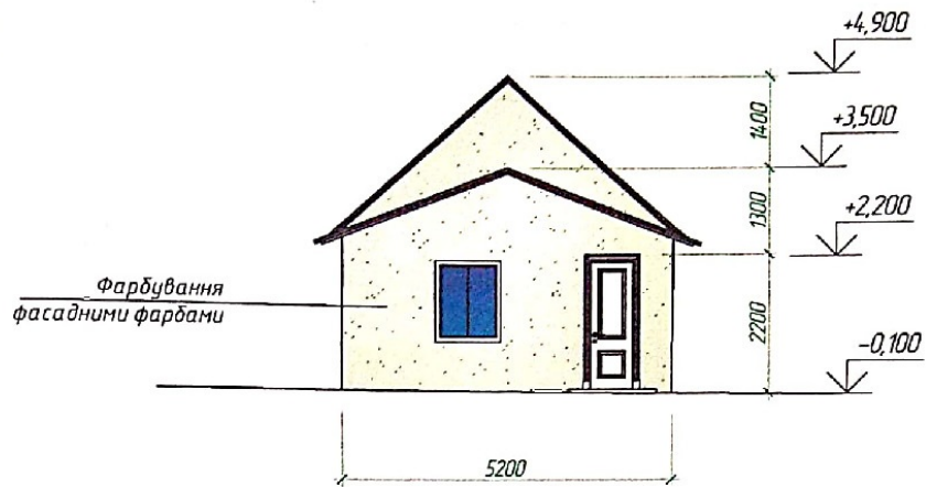
Фасад головний М 1:100.
